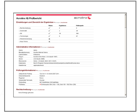
Detaillierter Prüfbericht
