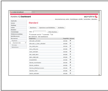
Lingware-Konfiguration
