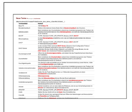
Neue Termvorschläge
